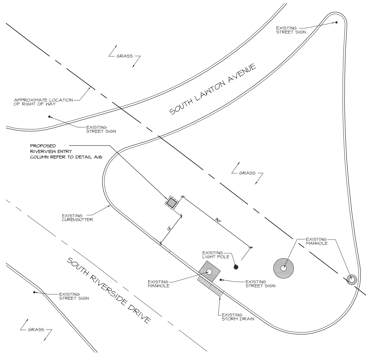
1 PLAN: INTERSECTION OF S. LAWTON AVE. & S. RIVERSIDE DR. SCALE: 1" = 10'-0"
