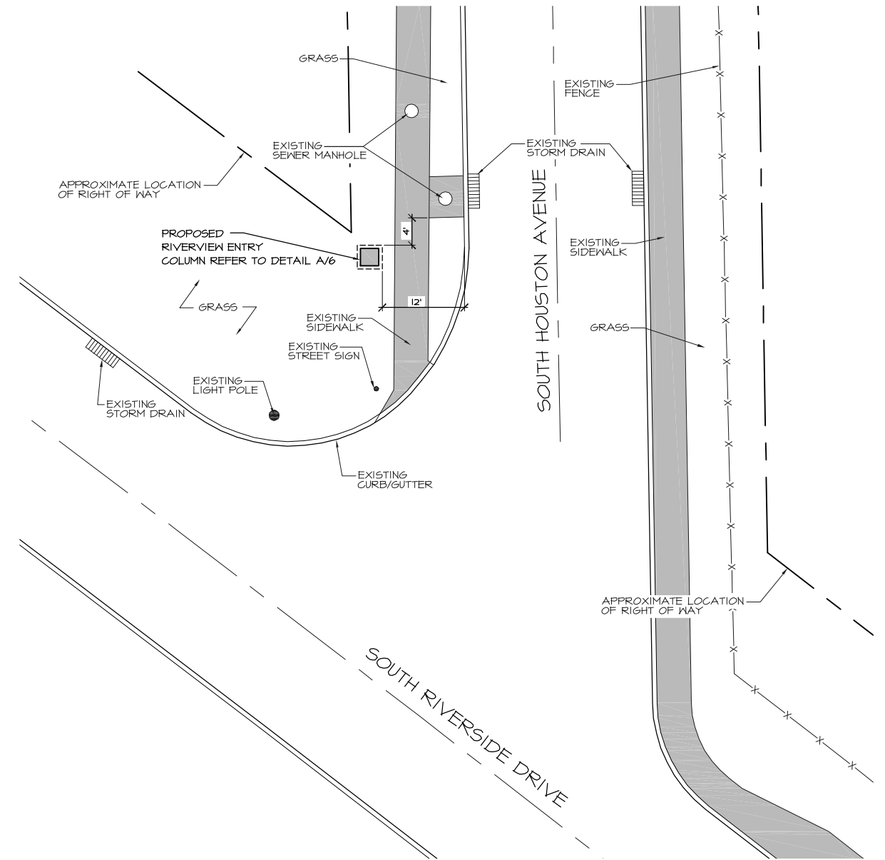
2 PLAN: INTERSECTION OF S. RIVERSIDE DR. & S. HOUSTON AVE. SCALE: 1" = 10'-0"
